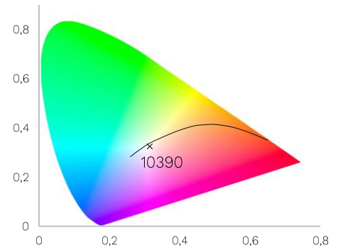
CRI (R1-R8) Farbwiedergabe nach Farben
