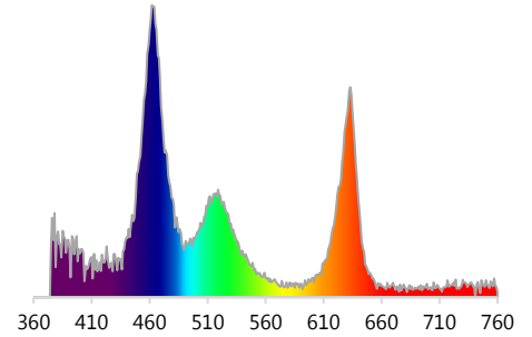
RGB Farbraum nach CIE 1931
